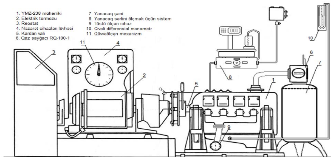
Şək. 1. Yeni fraksiya tərkibli nanokompozit alternativ dizel yanacağının motor sınaqlarının keçirilməsi üçün eksperimental stend
