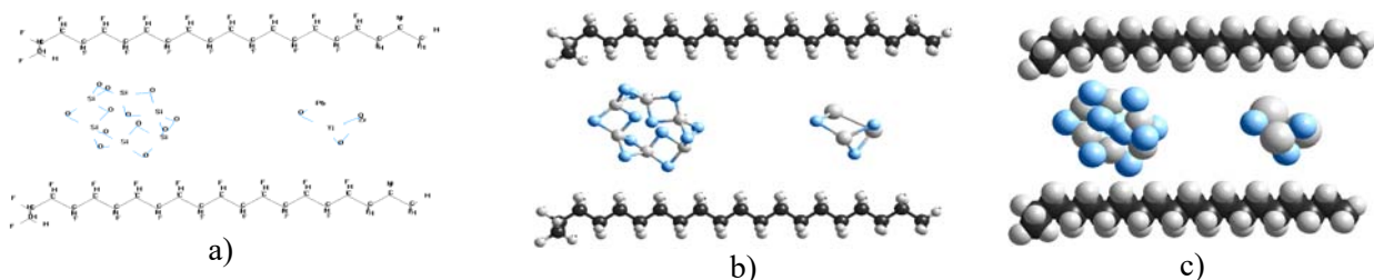
Şək. 3. PVDF 2(h-(-chf-chf-)10-h)-(SiO 2 ) 6 -PbZrTiO 3 nanokompozitinin nəzəri modelləri: xətlə (a), xətt və kürelərlə (b), kürelərlə (c)
