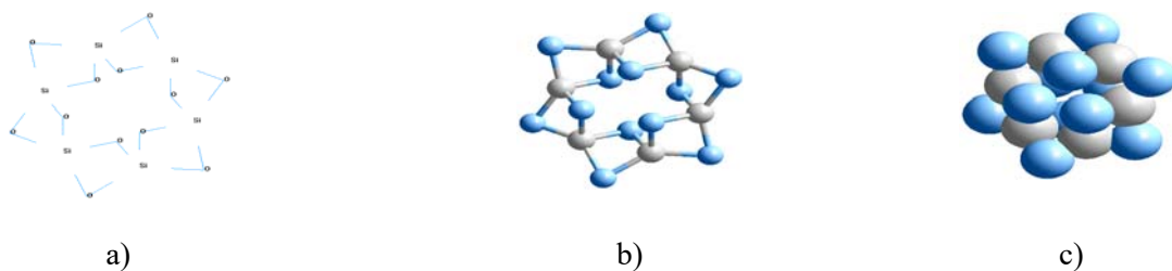
Şək. 1. (SiO 2 ) n nanohissəciyinin nəzəri modelləri (n=6, N=18): xətlə (a), xətt və kürelərlə (b), kürelərlə (c)
