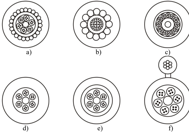
Şək. 5. Fiberoptik kabellərin nüvələrinin konstruksiyaları
