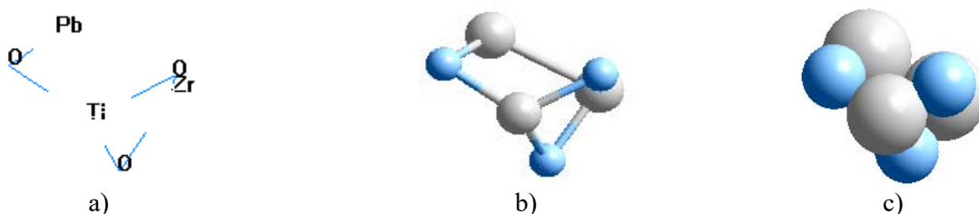
Şək. 2. Pb(ZrTiO 3 ) modelləri: xətlə (a), xətt və kürelərlə (b), kürelərlə (c)
