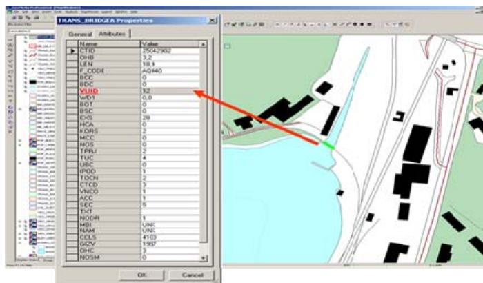
Şək. 2. Topoqrafik məlumat bazasının elektron xəritəsi və təfsilatlar cədvəli
