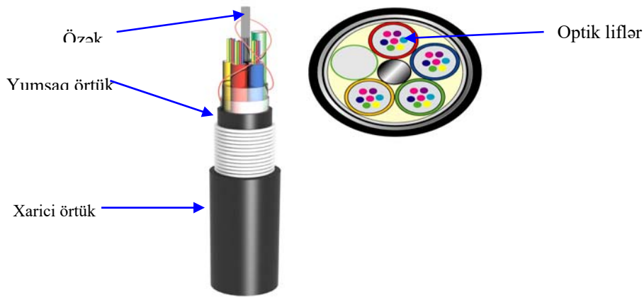
Şək. 2. Fiberoptik kabelin ümumi görünüşü
