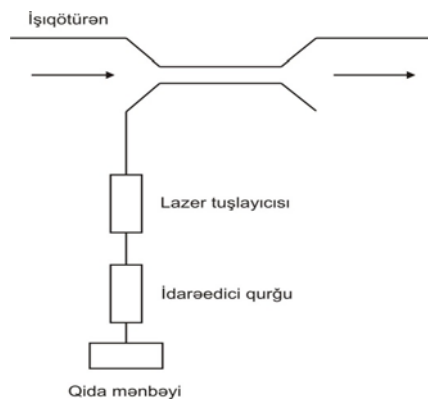
Şək. 5. Optik gücləndiricinin struktur sxemi
